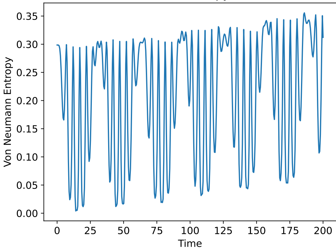
Von Neumann Entropy vs. Time
